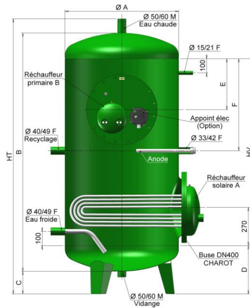
Version double échangeur
