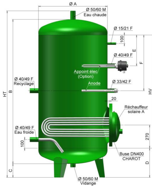
Version simple échangeur
